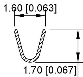
SECTION: A-A SCALE: 1:1
