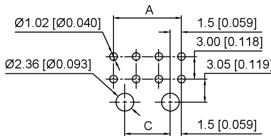
P.C.B LAYOUT: TOP VIEW Ploes: 2x04~2x12
