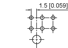
P.C.B LAYOUT: TOP VIEW Ploes: 2x03
