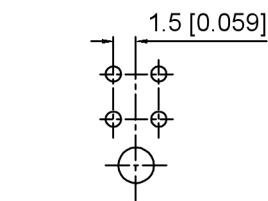
P.C.B LAYOUT: TOP VIEW Ploes: 2x02
