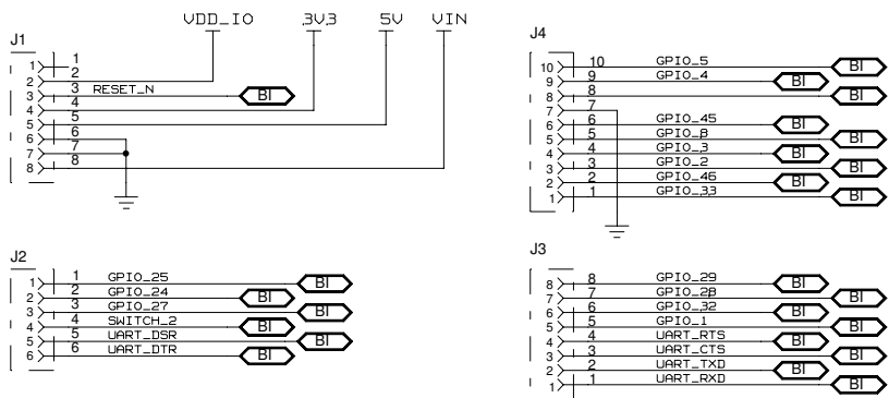
ARDUINO INTERFACE
