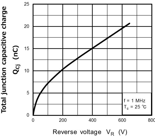
Fig. 8.5 Q_{cj} - V_R
