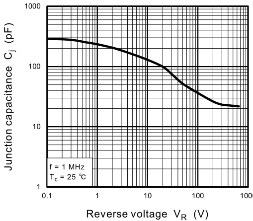
Fig. 8.4 C_j - V_R (Per Leg)
