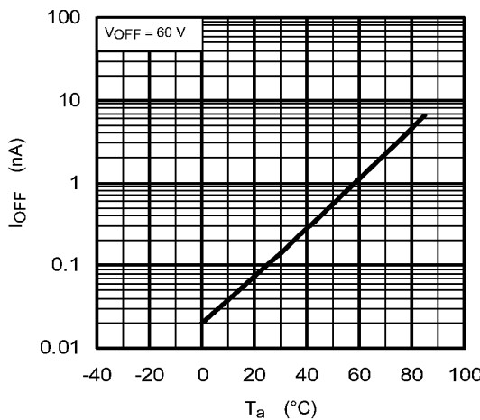
Fig. 14.9 I_{OFF} - T_a
