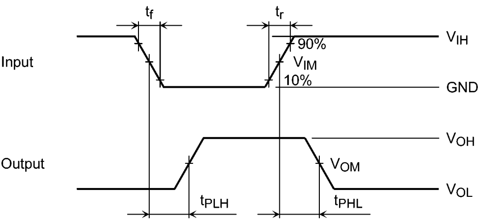
Fig. 12.8.1 t_{PLH} , t_{PHL}
