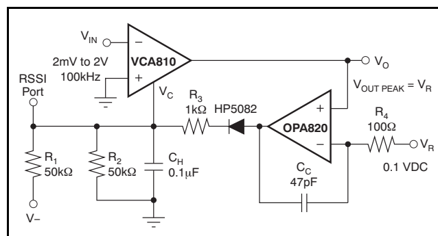
Figure 32. 60dB Input Range AGC
