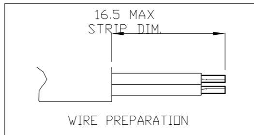
N°4 RECEPTACLE CONTACTS P/N 166051-1
