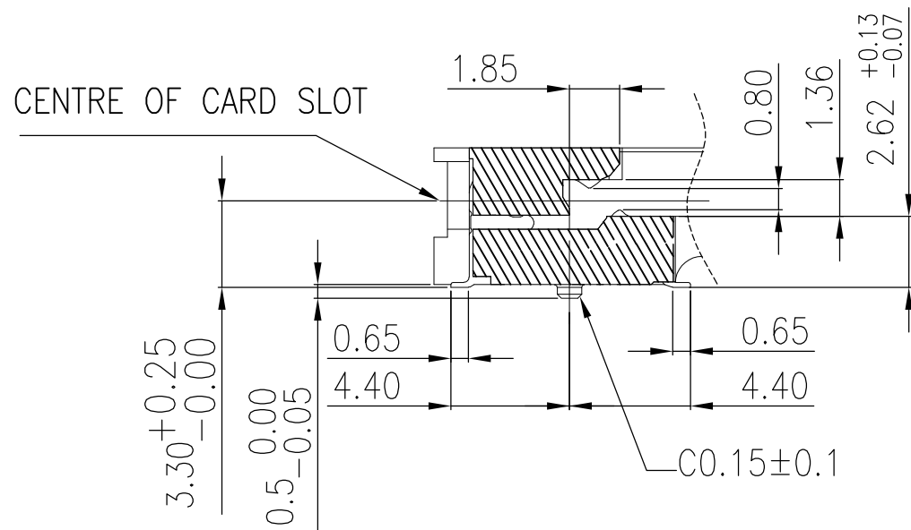
SECTION:A-A SCALE 2:1
