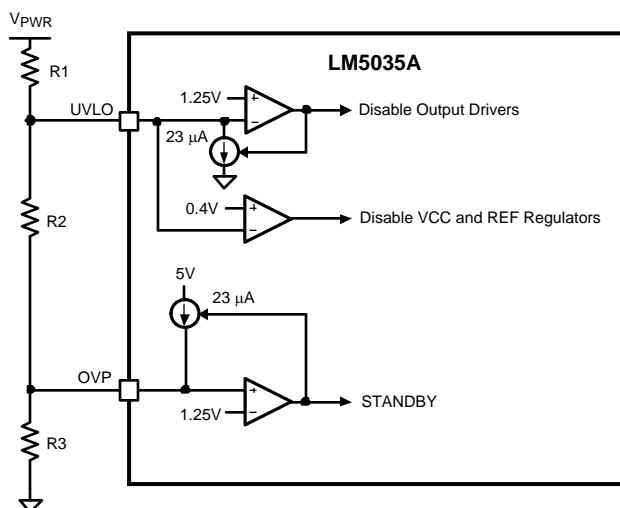
Figure 24. UVLO/OVP Divider
