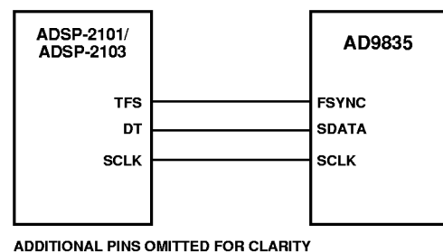
Figure 24. ADSP-2101/ADSP-2103-to-AD9835 Interface
