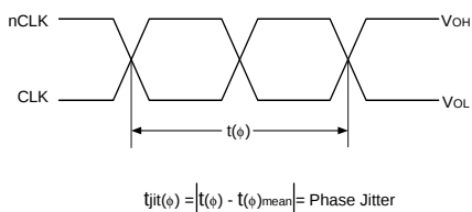
PHASE JITTER
