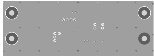
Inner1 Layer
