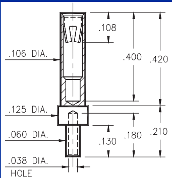
8730-0-19-XX-23-XX-10-0 Wire Termination
