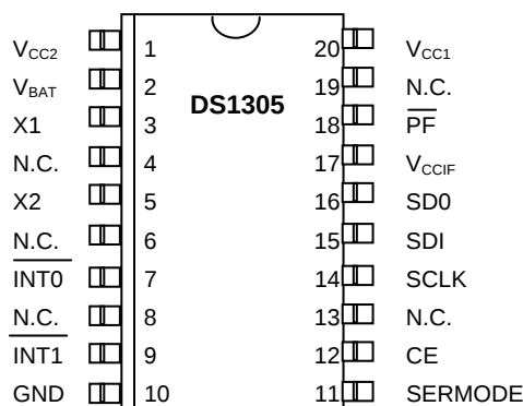
TSSOP (4.4mm)
