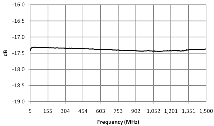
Coupling (Pin6-4)
