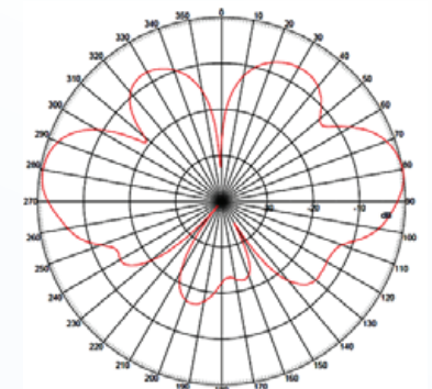
E-plane 1.92 GHz
