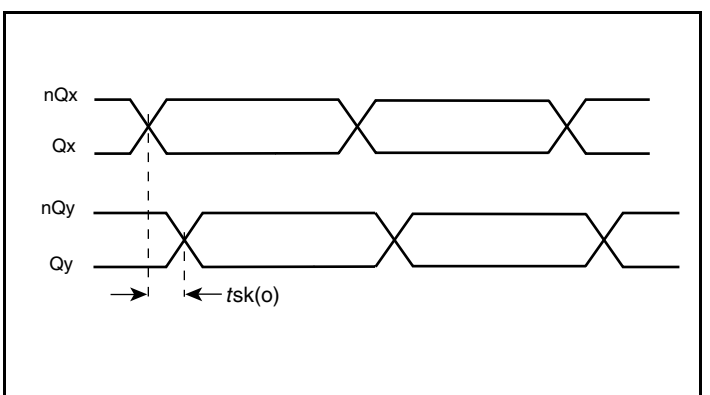
Output Skew
