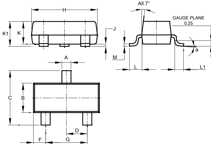
SOT23
