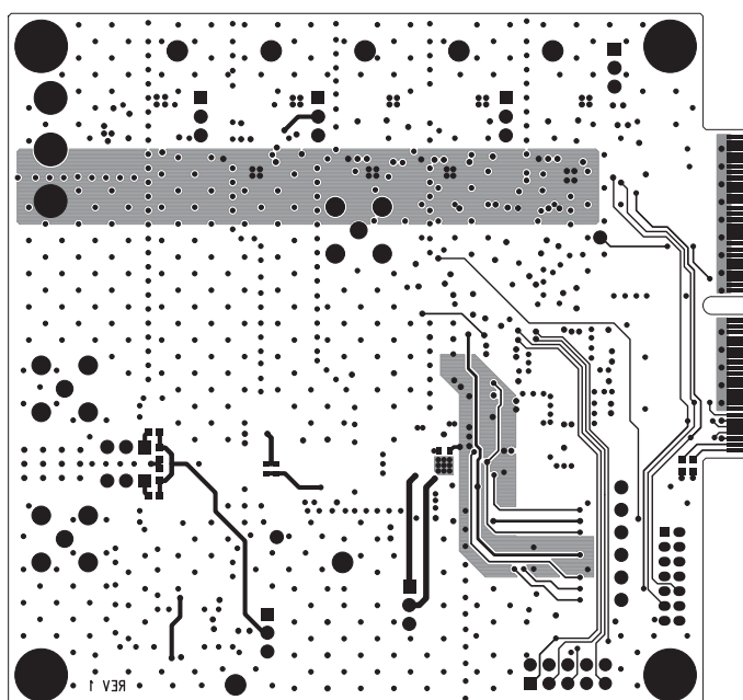
Layer 4 Bottom Layer
