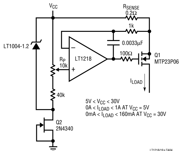
LT1218/19 • TA04
