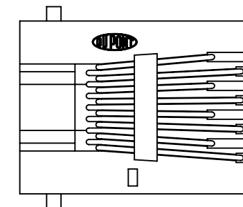
VIEW A-A
